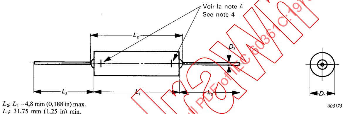
FIG. 2. — Dimensions pour le type 3.A.2. Dimensions for type 3.A.2.
