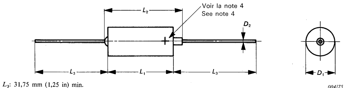
FIG. 1. — Dimensions pour le type 3.A.1. Dimensions for type 3.A.1.
