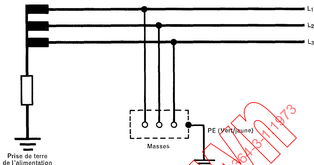
FIG 5 — Schéma IT
