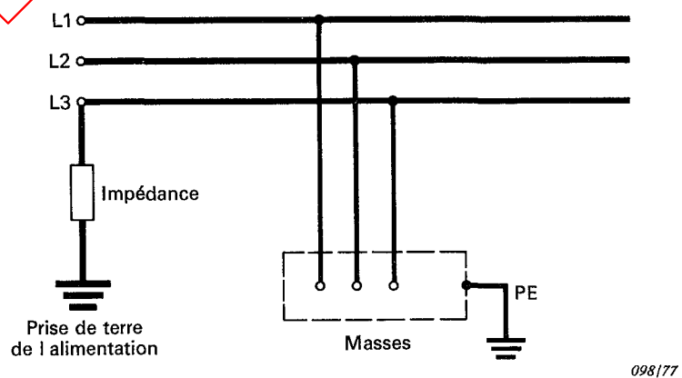
FIG 31E – Schéma IT
