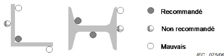
Figure 44.R21 – Emplacement des câbles dans des éléments de construction métallique
