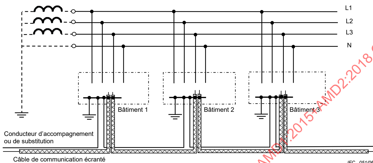
Figure 44.R2 – Exemple de conducteur d'accompagnement ou de substitution en schéma TT
