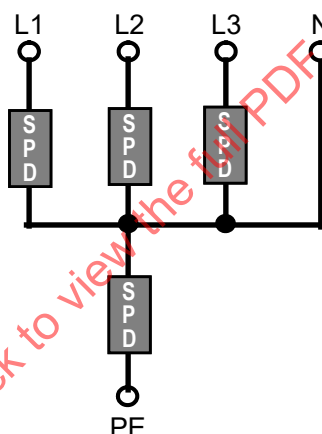
Figure 3 – Type de connexion CT1 (configuration 3+0) pour un réseau triphasé
