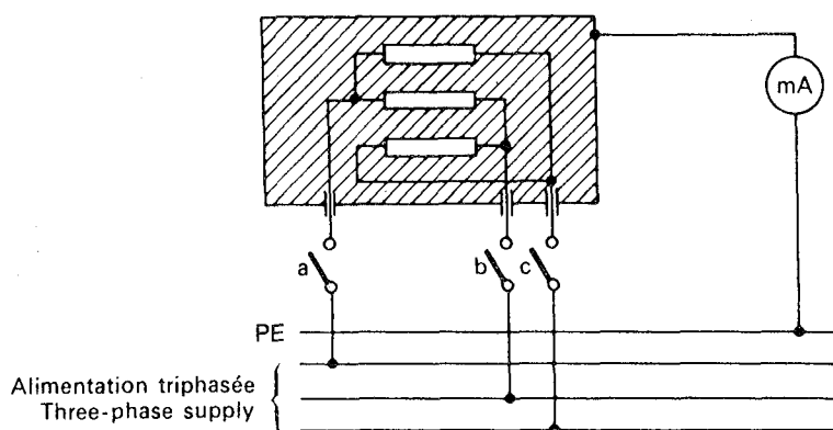
FIG. 5. — Schéma pour la mesure du courant de fuite à la température de régime pour connexion triphasée.
