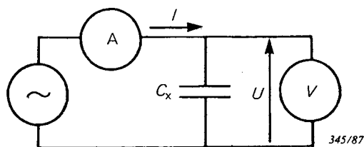
FIG. 1. — Schéma de principe du circuit de mesure de l'impédance.
