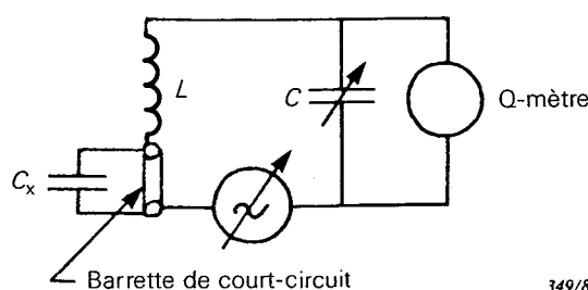
FIG. 6. — Schéma de principe du circuit de mesure.
