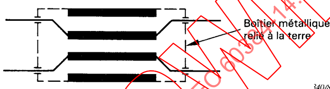
FIG. 3c. — Condensateur multiple de traversée (non coaxial) pour utilisation symétrique et asymétrique.
