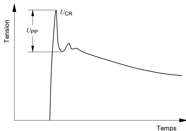
Figure 7 – Forme d'onde d'un choc
