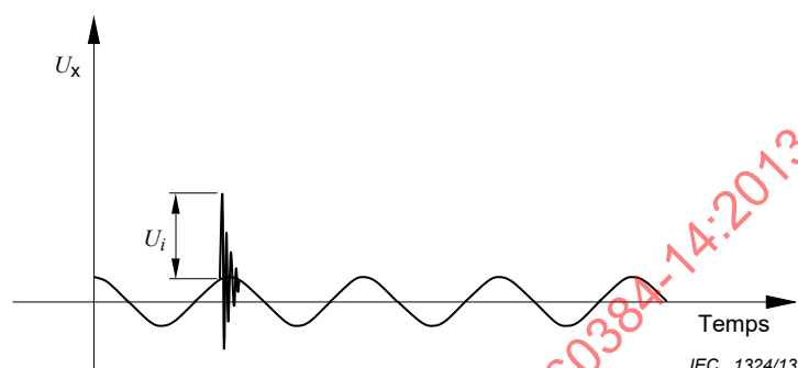
Figure 9 – Onde alternative fondamentale avec une impulsion haute tension superposée non synchronisée aléatoire
