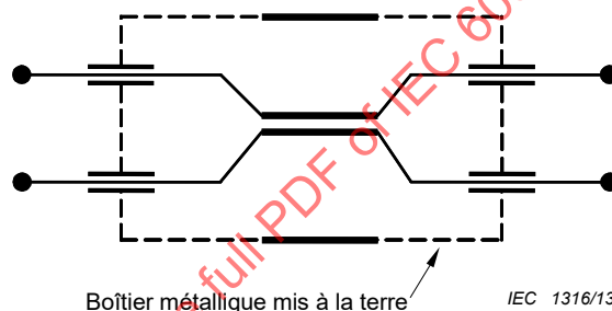
Figure 4c – Condensateur de traversée à plusieurs unités pour utilisation symétrique et asymétrique (non coaxial)
