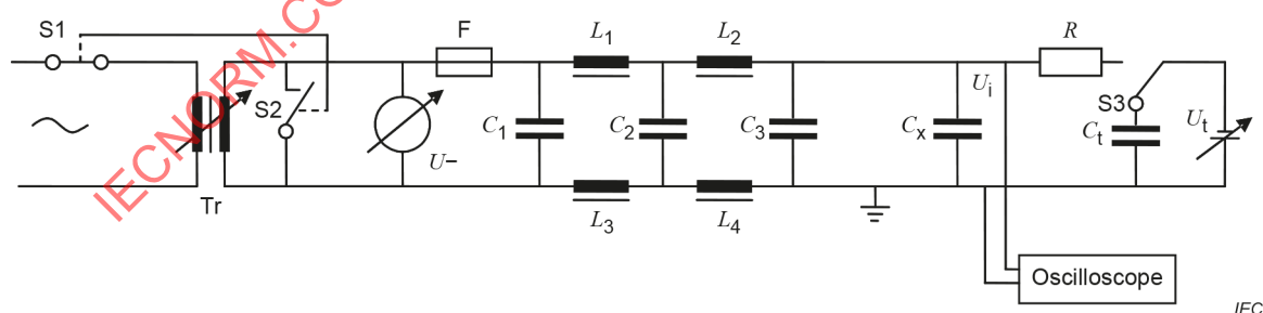
Figure 7 – Circuit typique pour charger en impulsions des condensateurs soumis à une tension alternative
