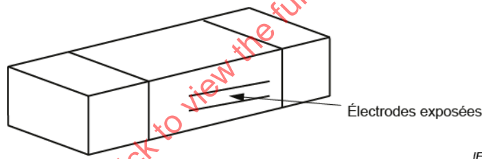
Figure 4 – Électrodes exposées
