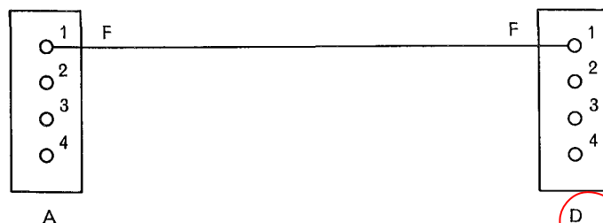
FIG. 6. — Exemple de repère de fonction.
