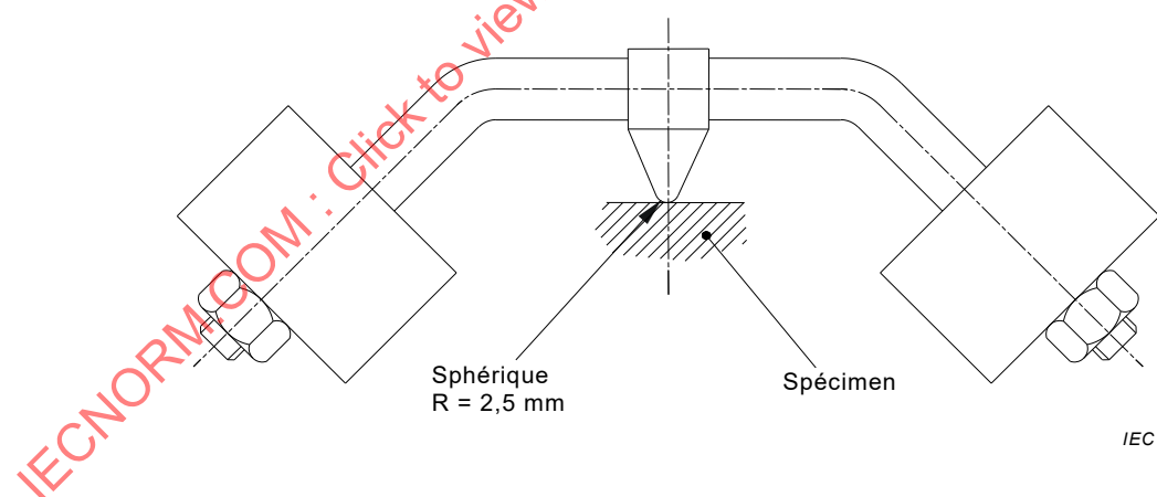
Figure 7 – Appareil pour l'essai à la bille
