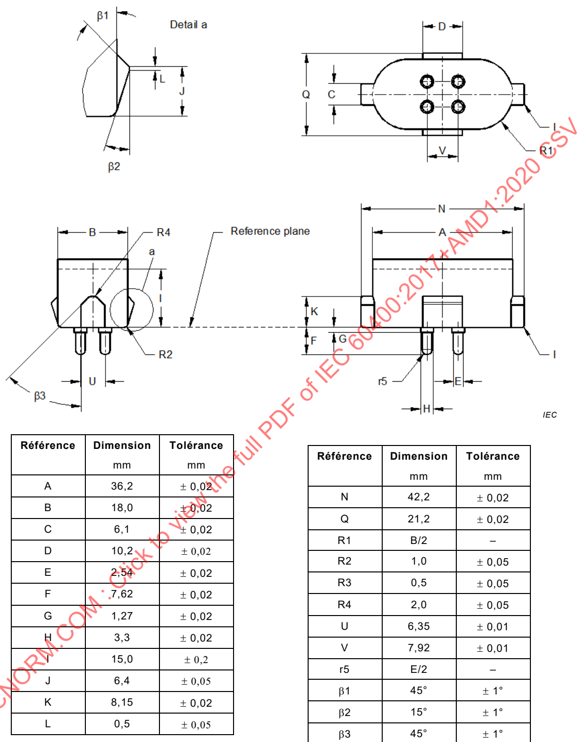
Figure 33 – Culot d'essai pour l'essai de 18.1 pour douilles GX10q
