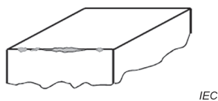
Figure 8 – Ragged edge
