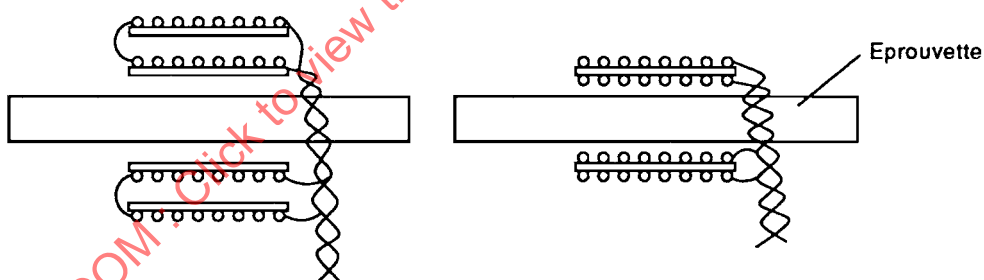
Figure 5c – Bobines de mesure du champ d'excitation (bobines de H) de type coaxial. La bobine intérieure et la bobine extérieure sont branchées en série opposition
