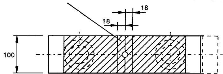
Figure 4a – Vue de côté
