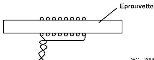
Figure 5a – Bobine de mesure de flux (bobine de B) enroulée autour de l'éprouvette
