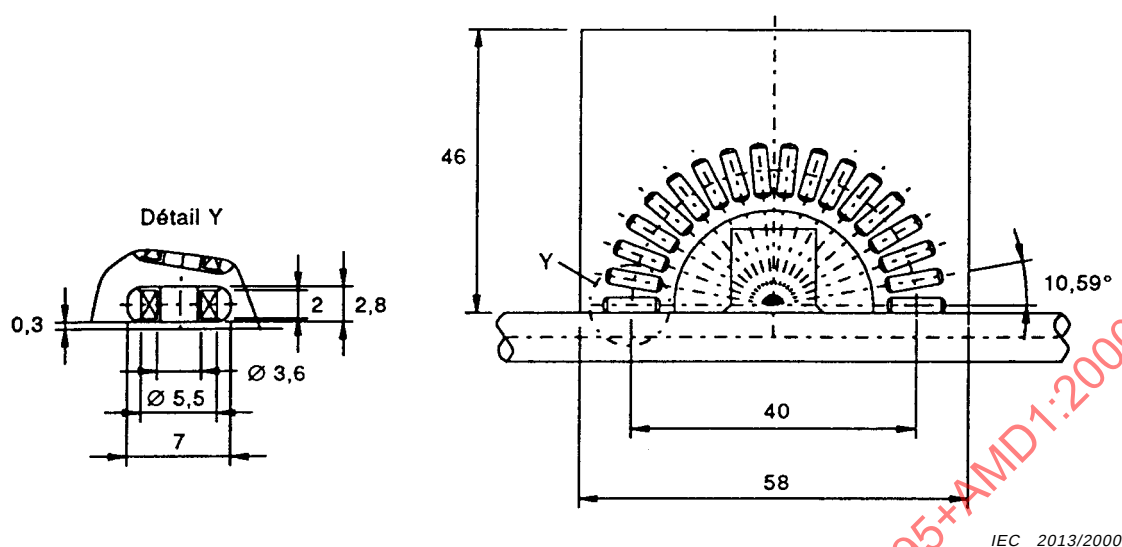
Figure 5e – Système de bobines séparées constituant un potentiomètre de Rogowski-Chattock pour la mesure de I
