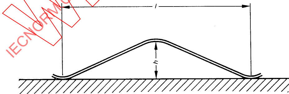
Fig. 2. - Facteur d'ondulation. Wave factor.
