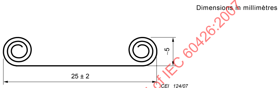
Figure 3 – Bande d'essai
