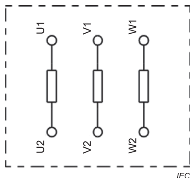
Figure 3 – Matériel triphasé à six bornes
