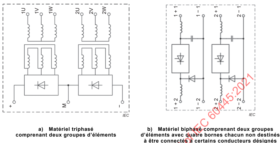
Figure 5 – Matériels à groupes d'éléments
