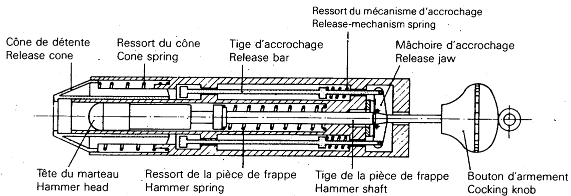
FIG. 2. — Appareil d'essai de choc. Impact-test apparatus.
