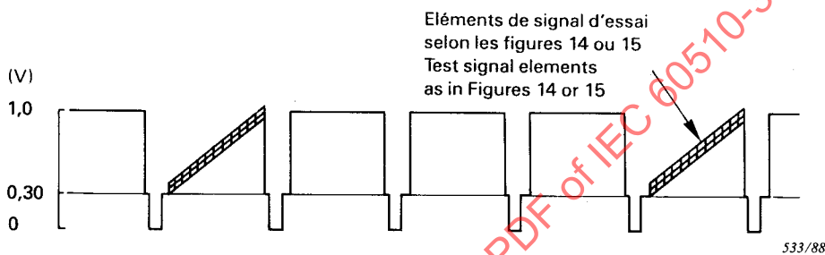
Fig. 7b. — Lignes intermédiaires au niveau du blanc. Composante moyenne d'image 87,5%. Intermediate lines at white level — 87.5% a.p.l.
