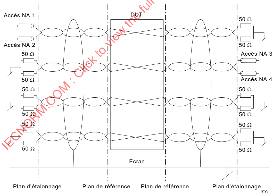
Figure 8 – Mesure de la télédiaphonie
