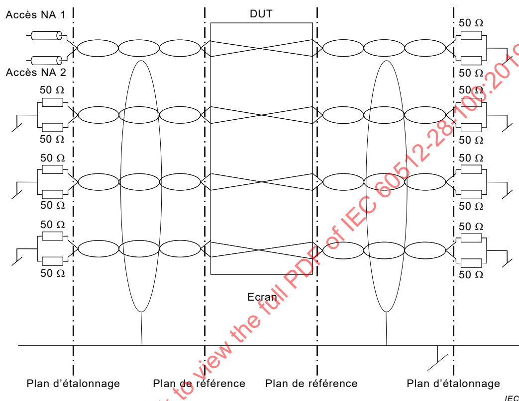
Figure 9 – Mesure d'affaiblissement de réflexion et de perte de conversion transverse (TCL)
