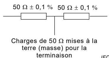
Figure 4 – Réseaux de charges résistives
