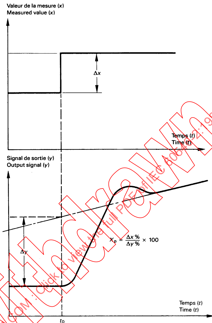
FIG. 3. — Courbes enregistrées au cours de l'essai de l'action proportionnelle. Recorded characteristics of proportional action.
