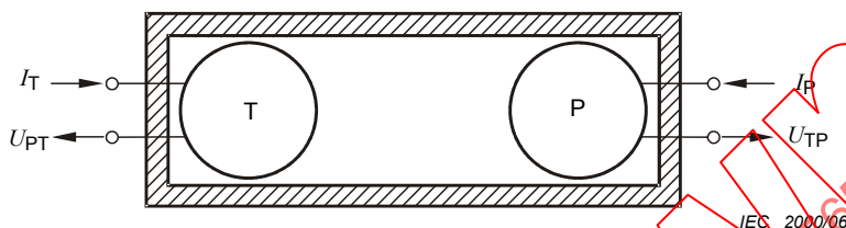
Figure 7 – Coupleur de référence avec deux transducteurs: un projecteur P et un transducteur réciproque T
