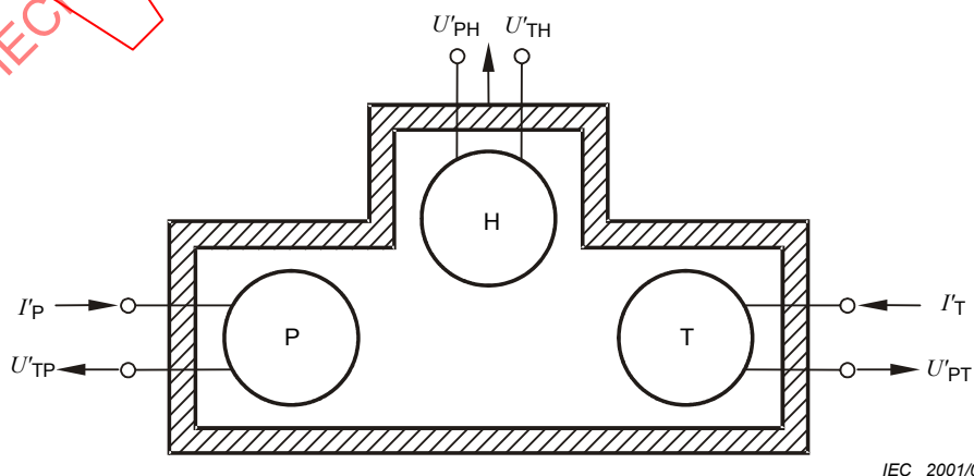
Figure 8 – Coupleur auxiliaire avec trois transducteurs: un projecteur P, un transducteur réciproque T, et un hydrophone H à étalonner
