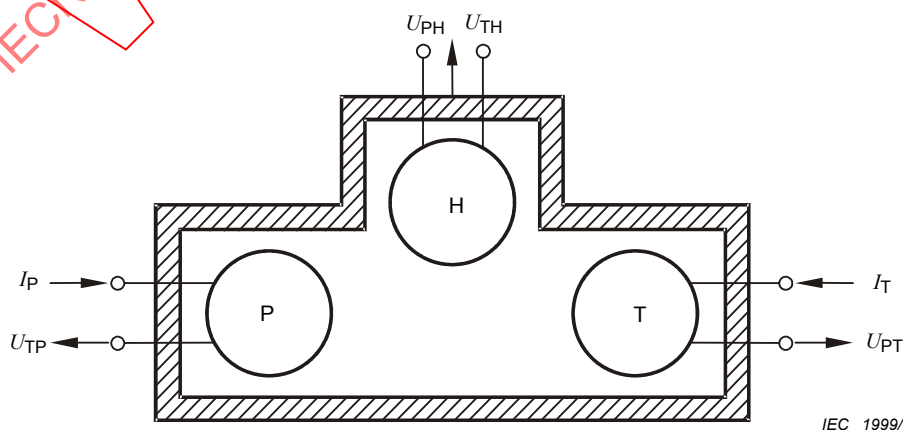
Figure 6 – Coupleur de réciprocité avec trois transducteurs; un projecteur P, un transducteur réciproque T, et un hydrophone H à étalonner
