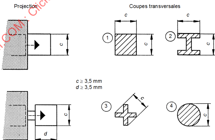
Figure 2 – Positions de mesure des contacts d'adaptateurs types de classe III
