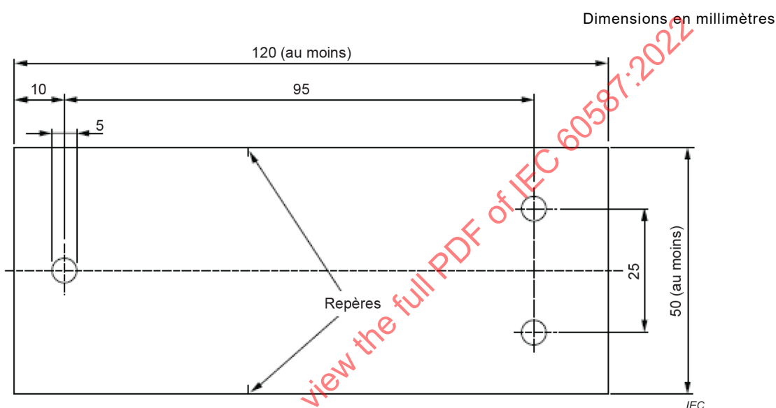
Figure 1 – Éprouvette à trous pour le montage d'électrodes
