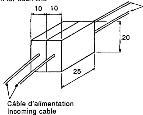
Figure 2 – Bloc de jonction pour essai de pose de luminaire à conducteurs de raccordement (sorties)
