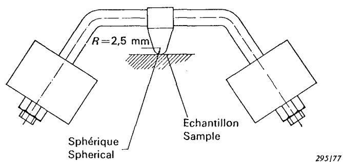
Figure 10 – Appareil pour l'essai de pression à la bille Ball-pressure apparatus
