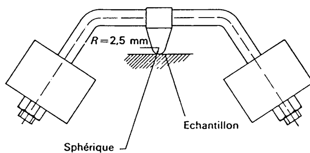
Figure 10 – Appareil pour l'essai de pression à la bille
