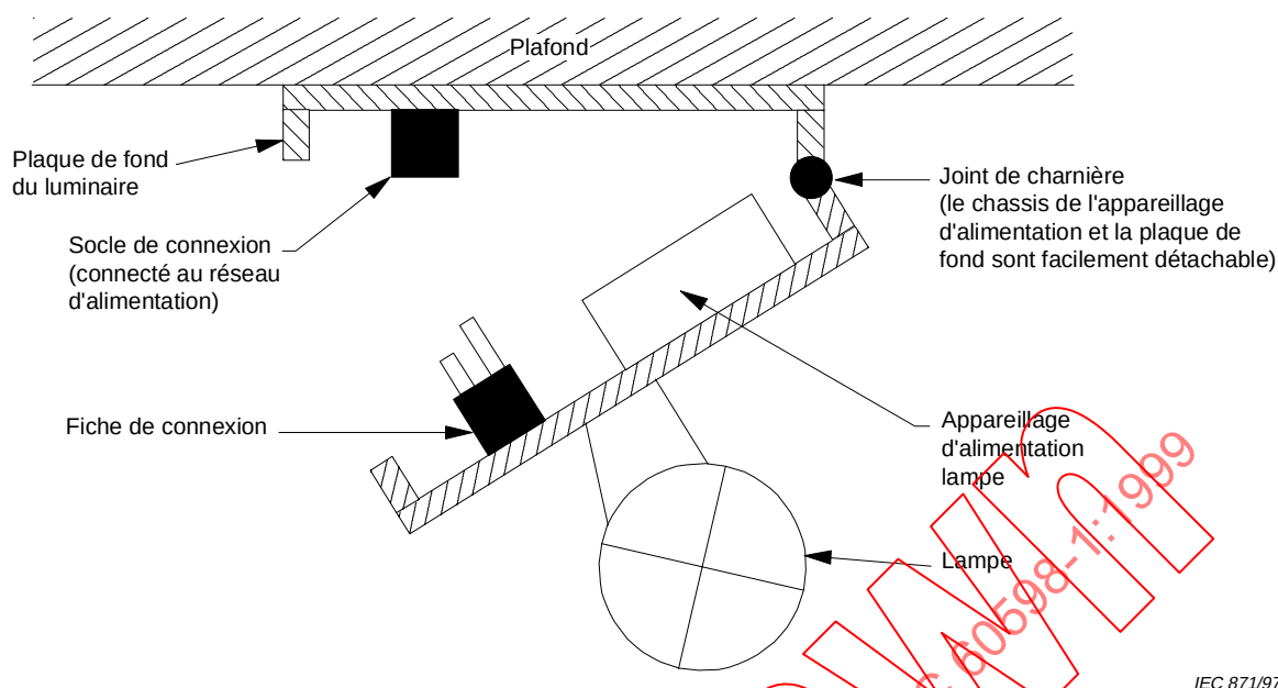
Figure FI 03 – Système de contact électromécanique avec connexion fiche/socle
