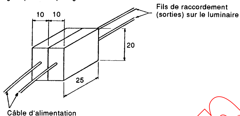
Figure 2 – Bloc de jonction pour essai de pose de luminaire à conducteurs de raccordement (sorties)
