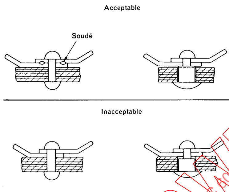
Figure 17 – Construction de connexions électriques
