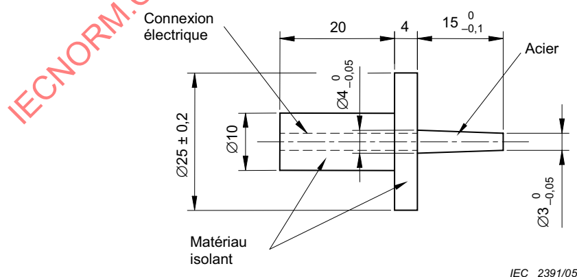
Figure 8 – Broche d'essai (voir 8.4.2 d) )
