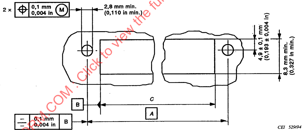
Figure 11 – Informations sur le montage des embases
