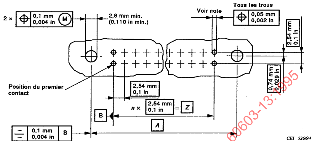
Figure 8 - Informations sur le montage des embases
