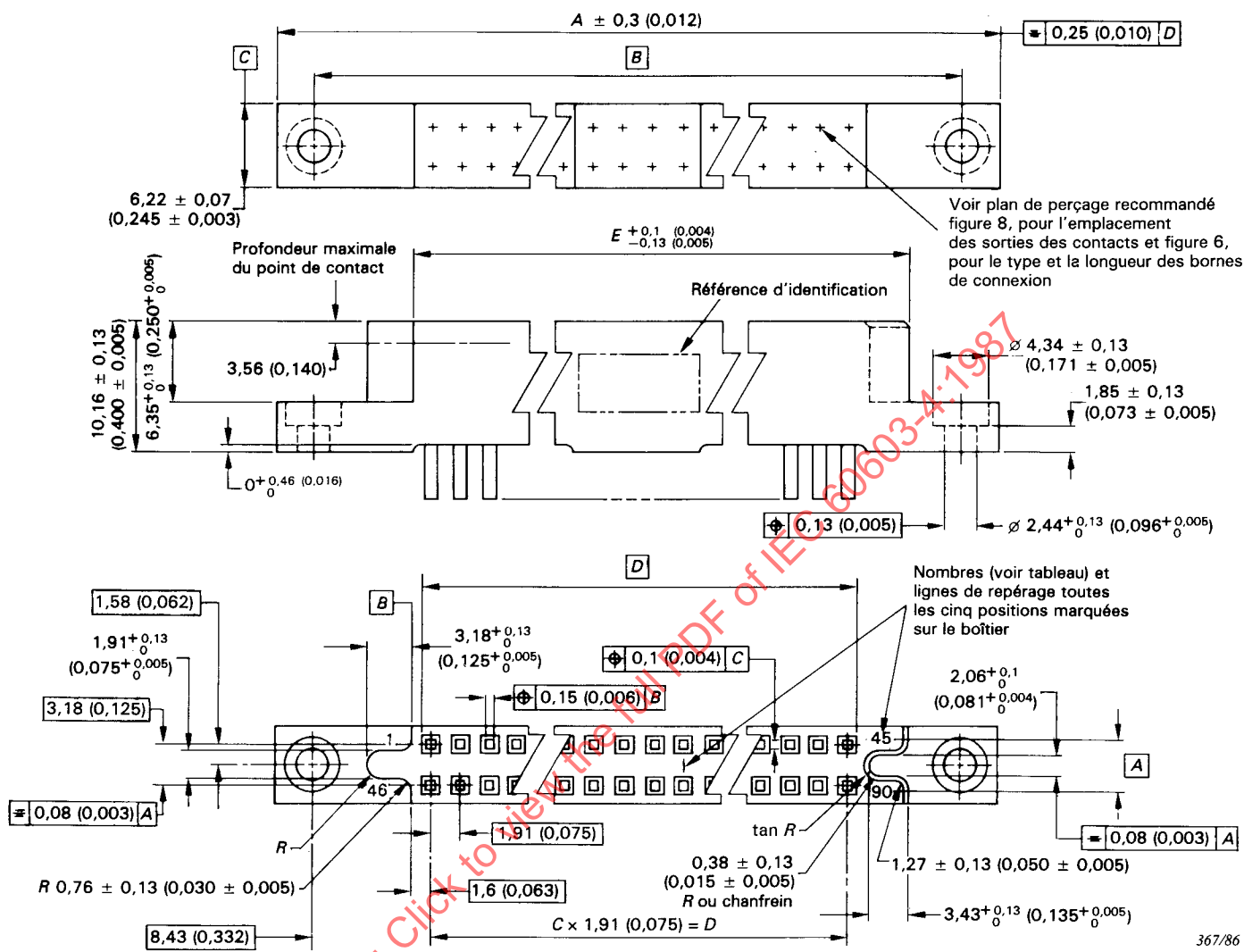
Dimensions en millimètres et en inches
