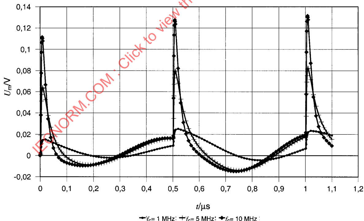
Figure D.5 – Réponse d'impulsion de DP pour une fréquence d'impulsion de DP considérée de 2 MHz pour différentes fréquences de coupure supérieure f_c du circuit d'essai; cela inclut un filtre coupe-bande de 3 ème ordre avec f_{centre} = 1 MHz [5] et [6]
