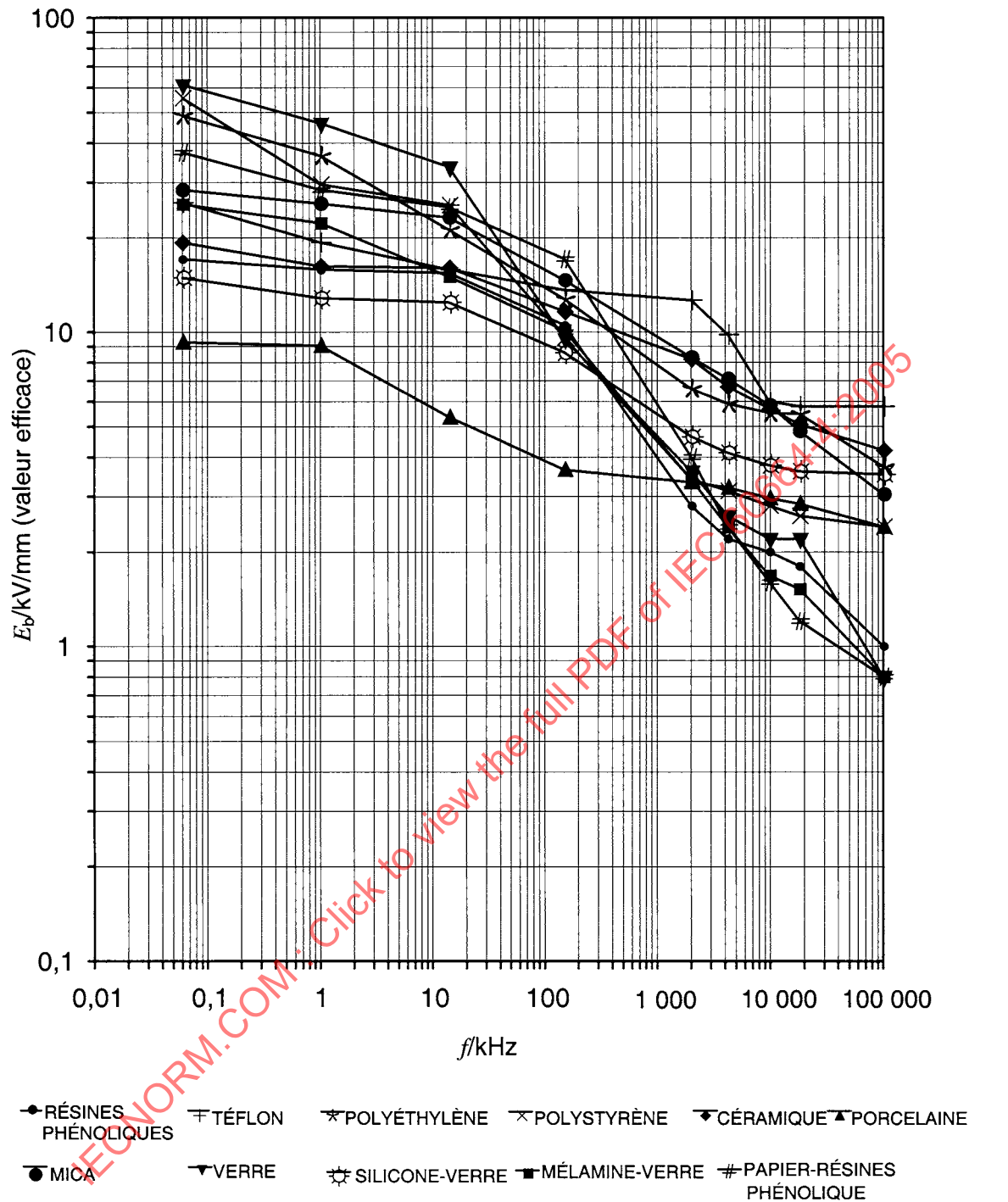
Figure C.3 – Claquage à haute fréquence, isolation solide; d = 0,75 mm [15]
