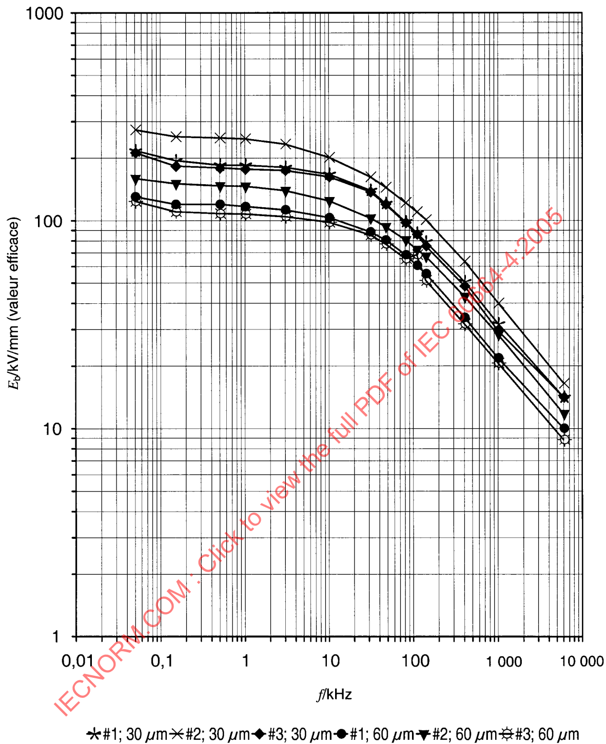
Figure C.5 – Claquage à haute fréquence, films isolants; #1: cellulose-acétobutyrate, #2: polycarbonate; #3: cellulose-triacétate [20]
