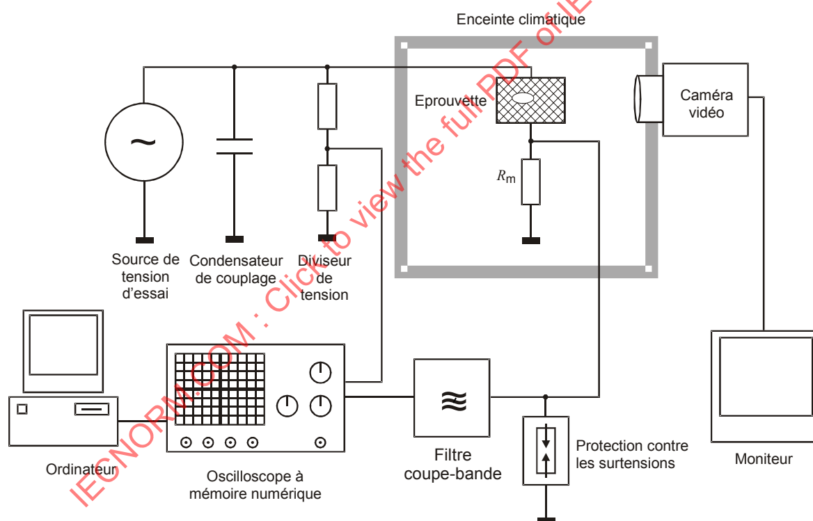
Figure D.4 – Schéma du circuit d'essai [5] et [6]
