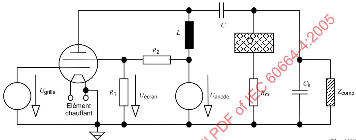
Figure D.2 – Oscillateur à puissance élevée et à haute fréquence [5] et [6]
