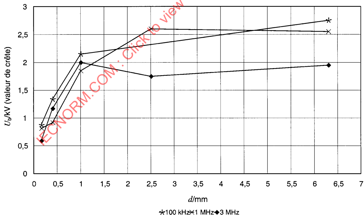
Figure B.2 – Résultats d'essai de la tension d'extinction de DP U_e des lignes de fuite jusqu'à 6,3 mm [6]
