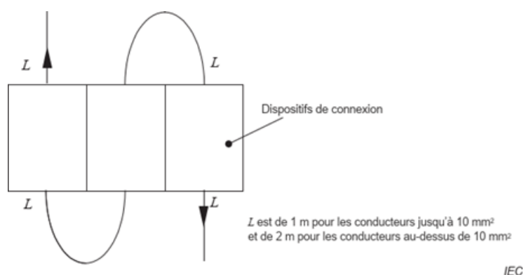
Figure 102 – Barrette de jonction
