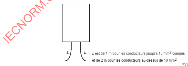
Figure 101 – Dispositif de connexion à une seule borne
