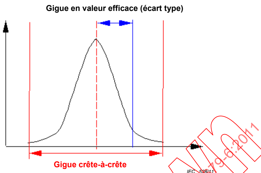
Figure 2 – Diagramme explicatif de la quantité de gigue appliquée à la gigue en valeur efficace
