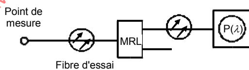
Figure 3 – Mesure de la longueur d'onde optique au moyen d'un coupleur MRL
