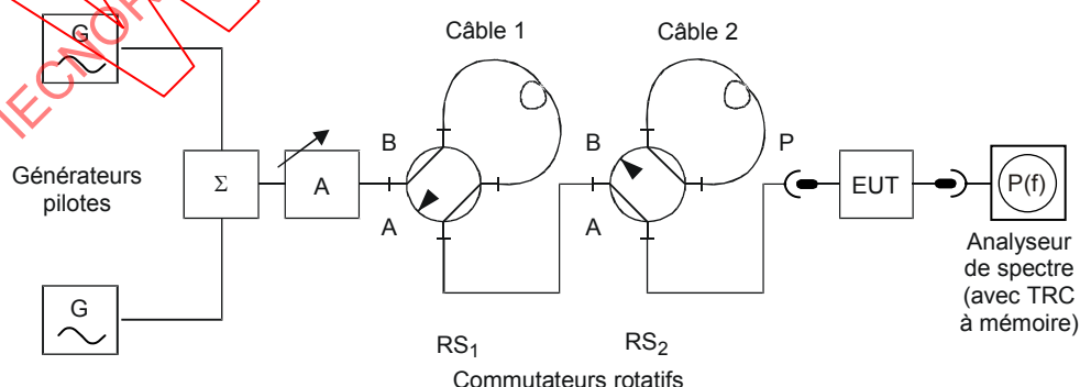
Figure 11 – Mesure de la réponse de la CAG à un échelon
