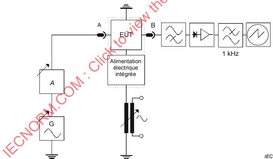
Figure 22 – Montage d'essai pour équipements à alimentation intégrée
