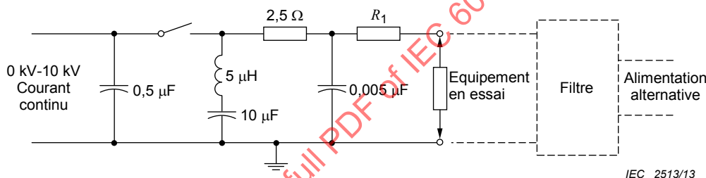
Figure H.4 – Schéma d'un générateur de transitoires oscillatoires 0,5 μs/100 kHz
