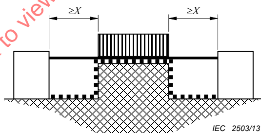
Figure B.5 – Partie non collée avec encoche étroite
