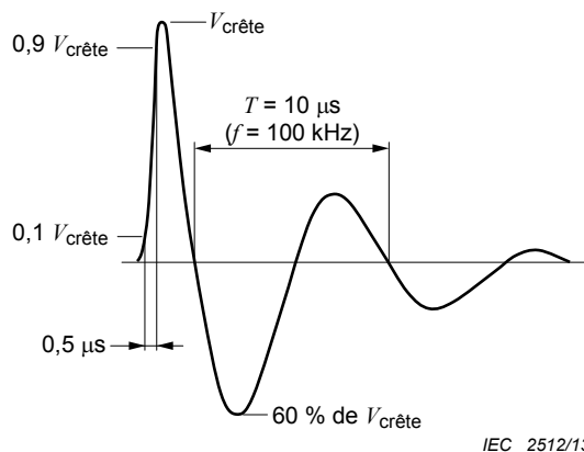
Figure H.3 – Caractéristiques d'un transitoire oscillatoire (tension en circuit ouvert)
