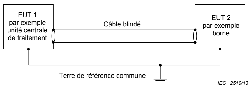
Figure R.1 – Exemple de protection contre les chocs électriques par blindage dans les bâtiments avec des systèmes de terre de référence commune
