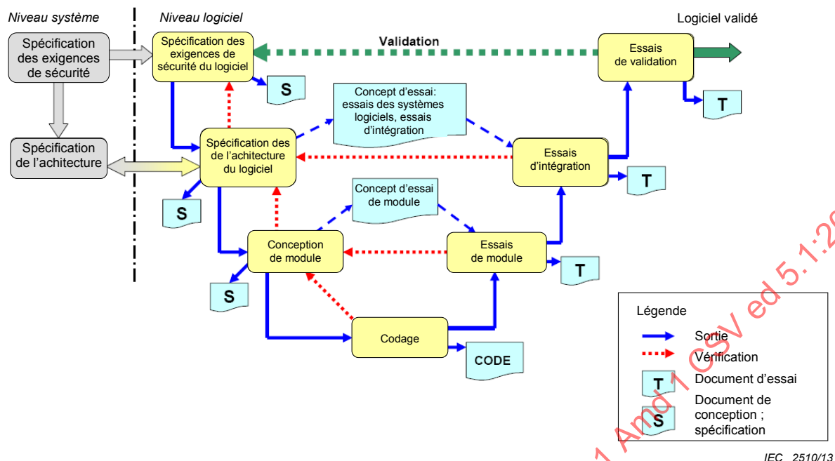
Figure H.1 – Modèle V pour le cycle de vie des logiciels
