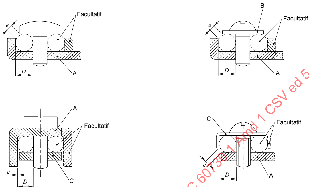
Bornes à serrage sous tête de vis
