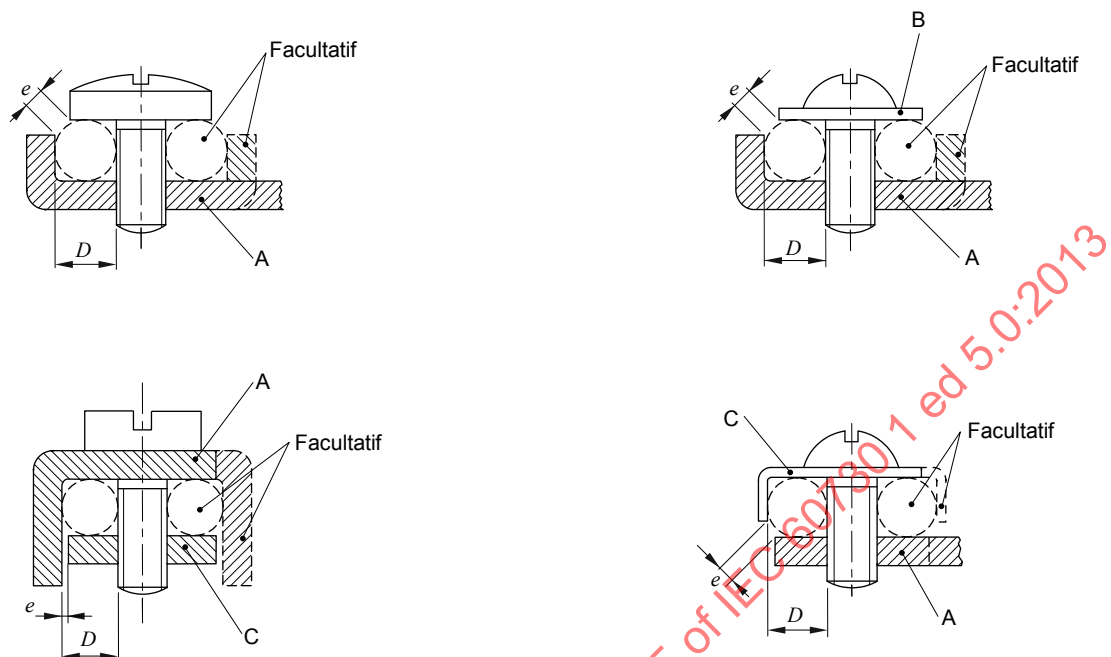
Bornes à serrage sous tête de vis
