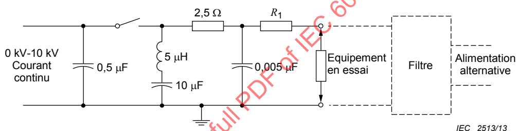
Figure H.4 – Schéma d'un générateur de transitoires oscillatoires 0,5 μs/100 kHz
