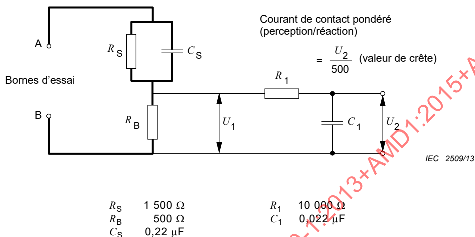
Figure E.1 – Circuit de mesure des courants de fuite
