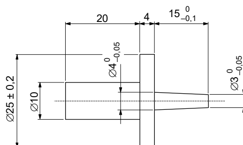
Figure 1 – Broche d'essai
