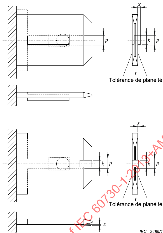
Figure 15 – Languettes pour des raccords non réversibles
