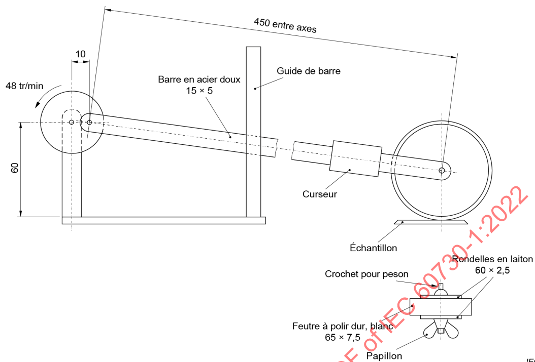
Figure 9 – Appareil pour vérifier l'indélébilité des marquages
