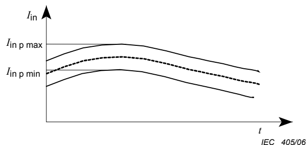
Figure 4 – I_{in} en fonction de t à U_{dc}
