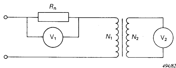
FIG. 2. — Mesures à champs faible et moyen.
