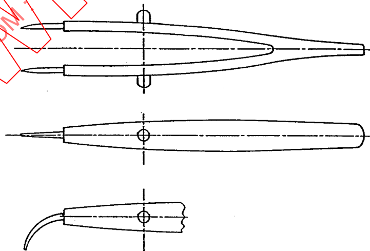
Brucelles – Tweezers
