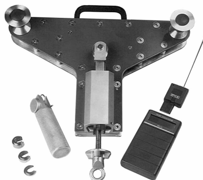
Différents modèles de dynamomètres — Different designs of dynamometers
