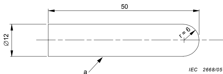
a) Détails du calibre d'essai
