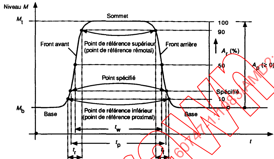
a) Impulsion dans le sens positif
