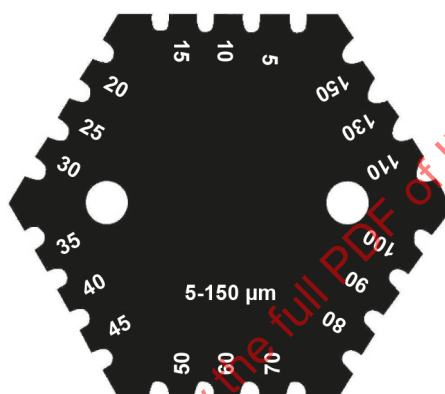
Figure B.1 – Exemple d'un calibre de mesure de l'épaisseur de la couche de pâte thermique isolante comprise entre 5 \mu\text{m} et 150 \mu\text{m}
