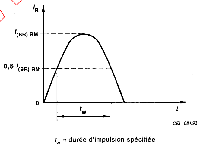
Figure 46 - Forme d'onde du courant inverse
