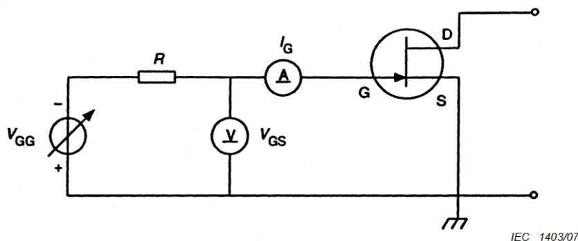
Figure 50 – Circuit de base pour la mesure de la tension de claquage grille-source V_{(BR)GSO}
