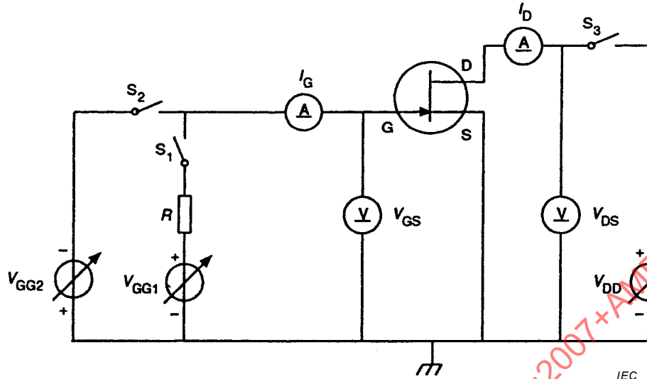
Figure 52 – Circuit pour la mesure de la résistance thermique canal-boîtier
