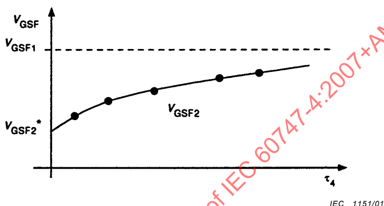
Figure 55 – V_{GSF2} en fonction du temps de retard \tau_4
